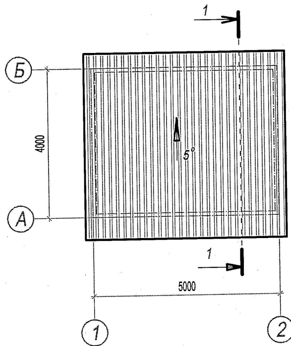
План покрівлі М 1:100
