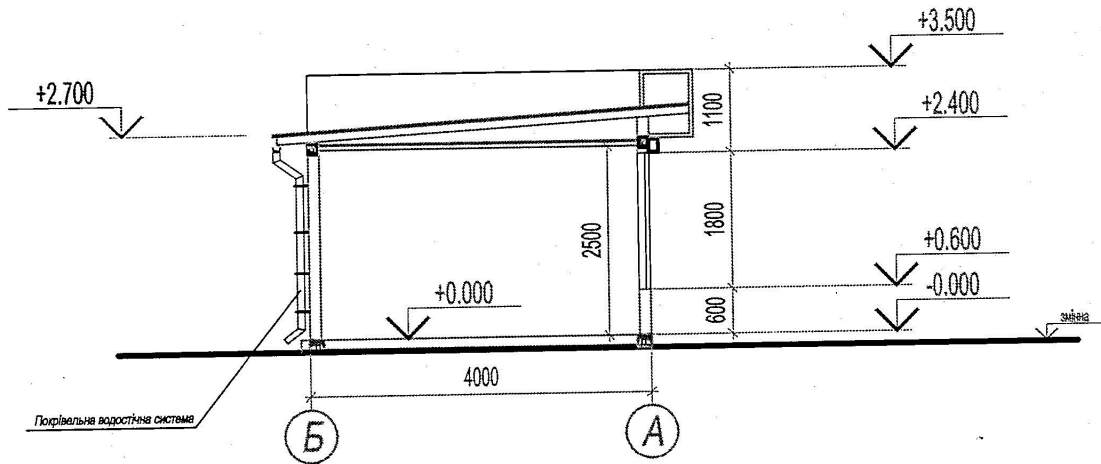
Розріз 1-1 М 1:100
