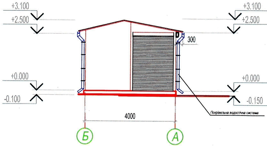
Фасад Б-А М 1:100
