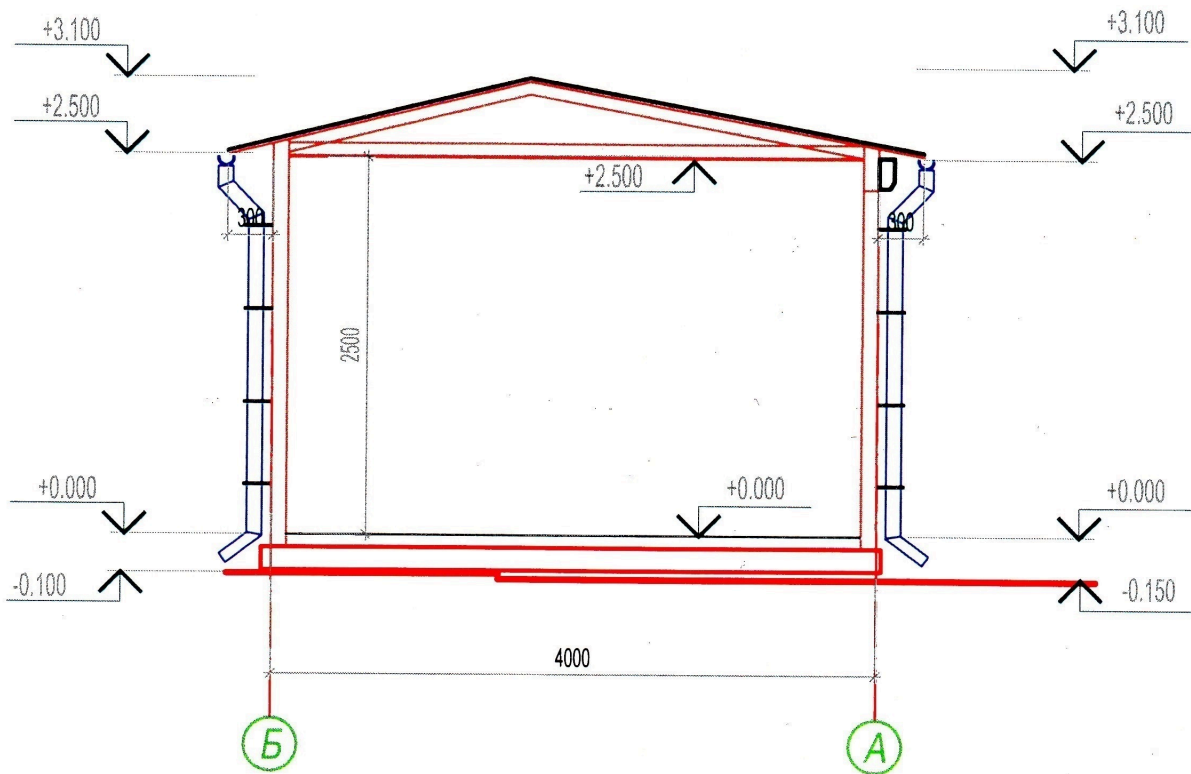
Розріз 1-1 М 1:50
