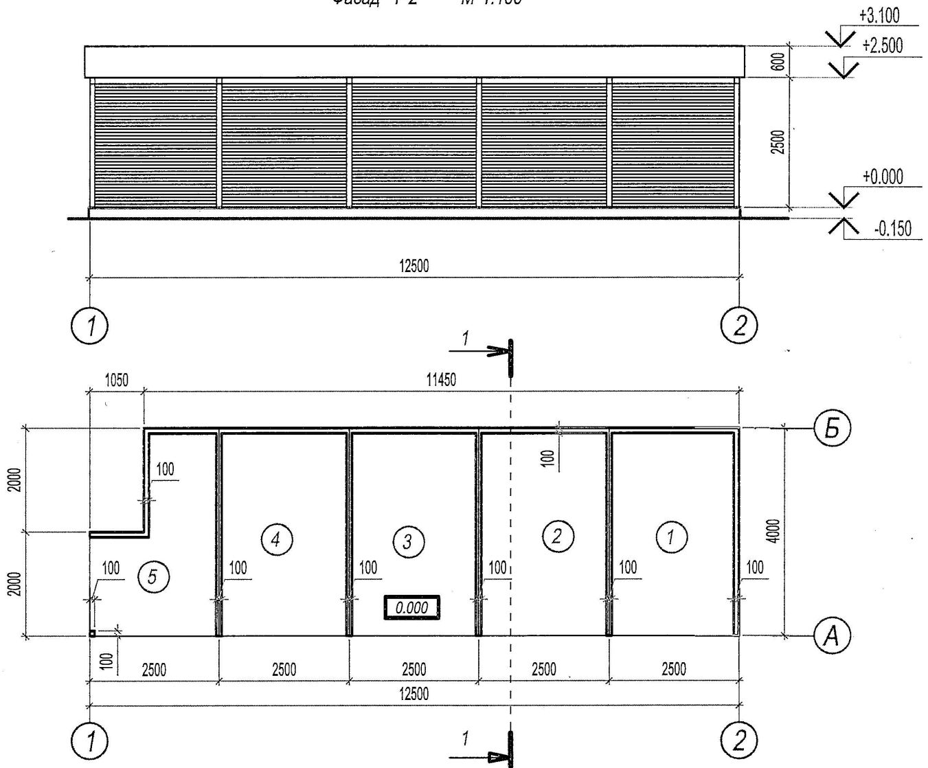
Фасад 1-2 М 1:100
